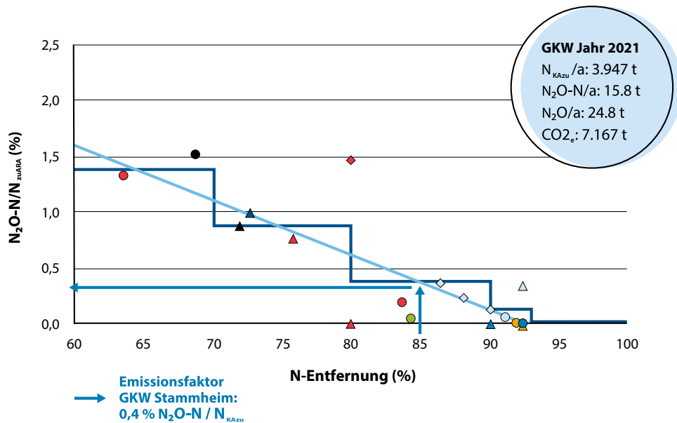
Abbildung 2: Emissionsfaktor N 2 O-N/N KAZU -KA in Abhängigkeit der N-Entfernung Quelle: nach Studie "ReLaKo" der TU Wien 2015 Die Studie untersuchte verschiedene Kläranlagen. Die unterschiedlichen Formen im Diagramm stellen die Ergebnisse der Kläranlagen dar.
