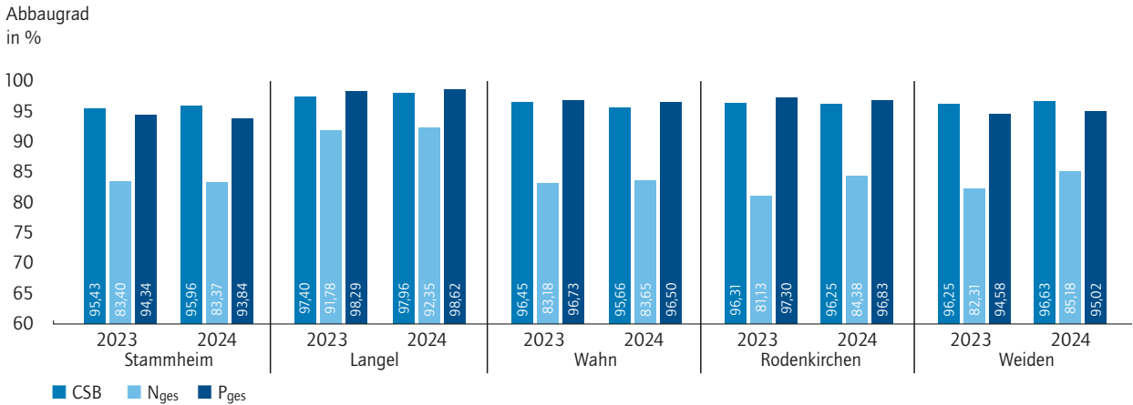
Abbildung 5: Abbaugrade der Kölner Klärwerke im Vergleich von 2023 und 2024
