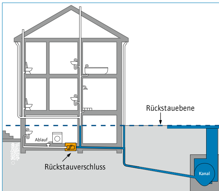
Abb. 38b – Rückstauverschluss | RICHTIG
