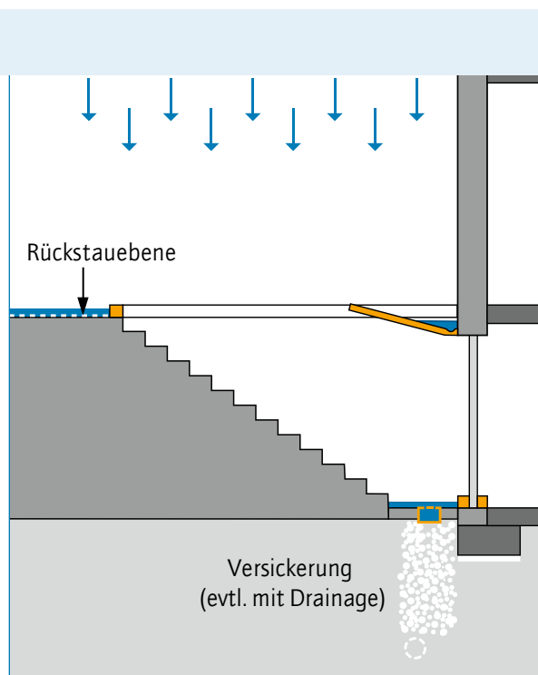
Abb. 19b – Kellertreppe | RICHTIG
