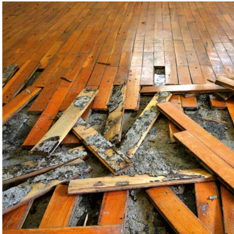
Abb. 48 – Schäden durch Stauwasser
