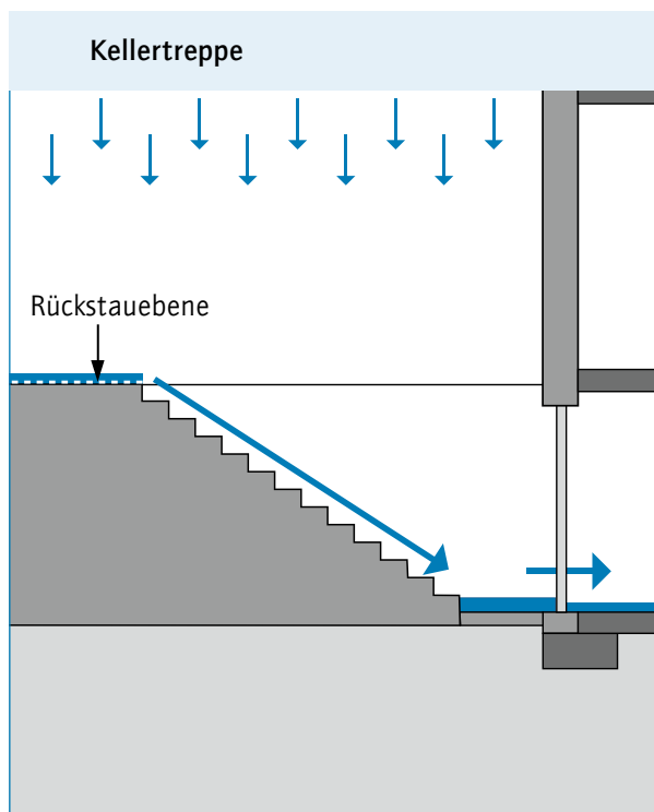
Abb. 19a – Kellertreppe | FALSCH
