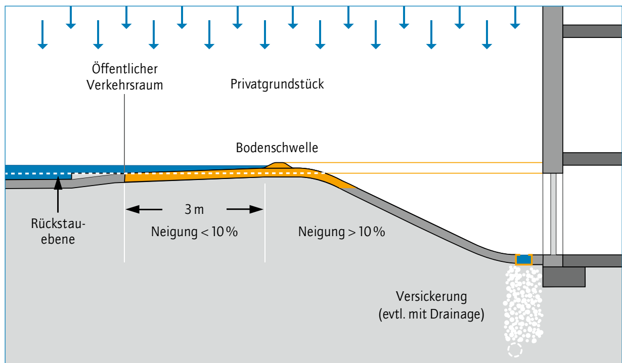
Abb. 18 – Bodenschwelle vor Tiefgaragenzufahrt
