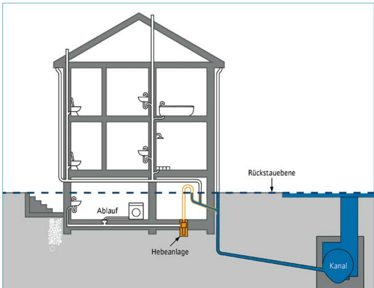
Abb. 40 – Hebeanlage
