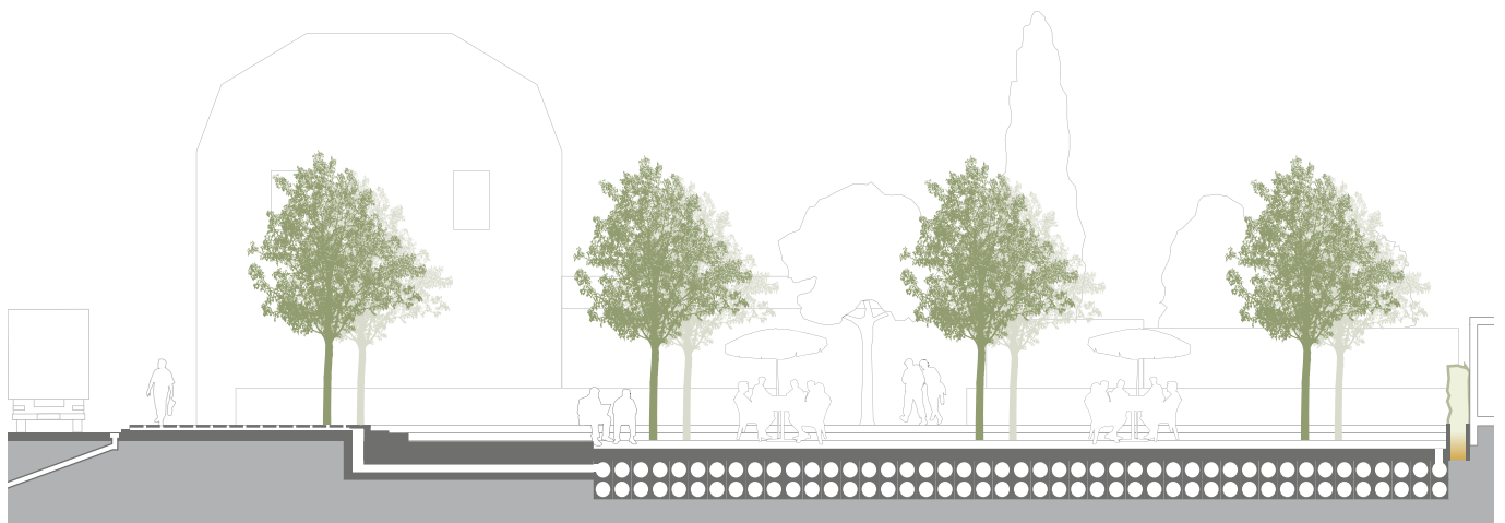
80 Parkplatz Schulstraße: Querschnitt Variante C
