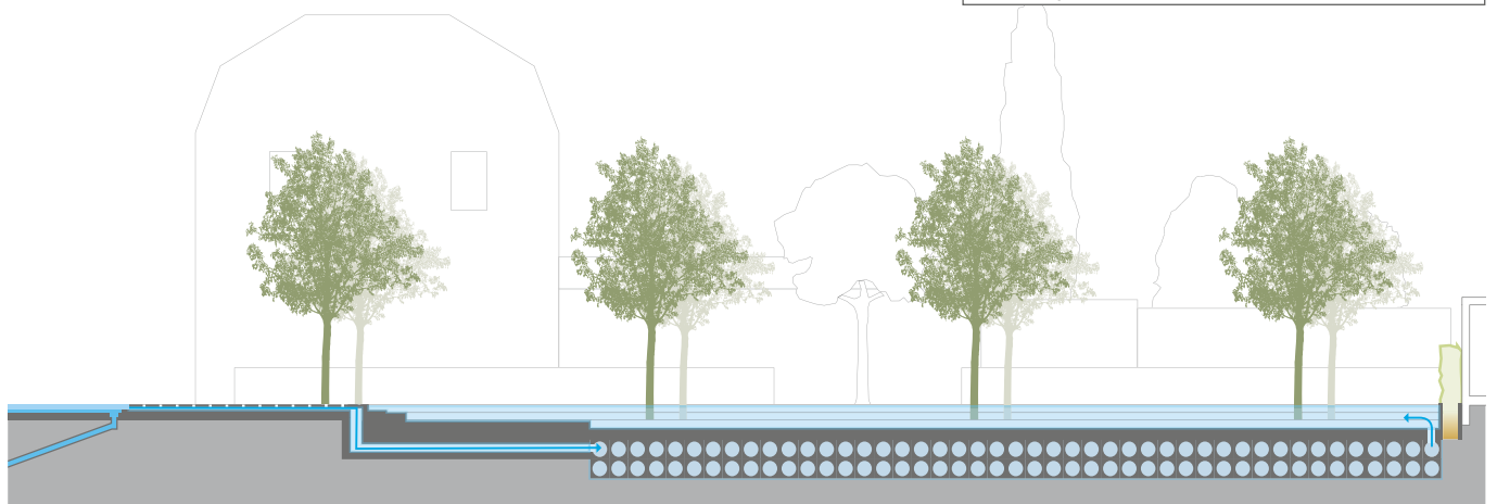
81 Parkplatz Schulstraße: Querschnitt Variante C nach einem starken Regenereignis
