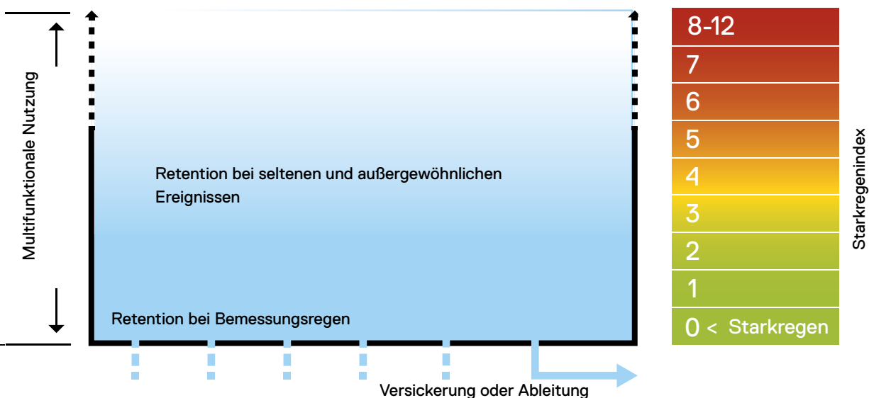
06 Typ 2 – Retentionsraum mit regelmäßiger Beschickung
