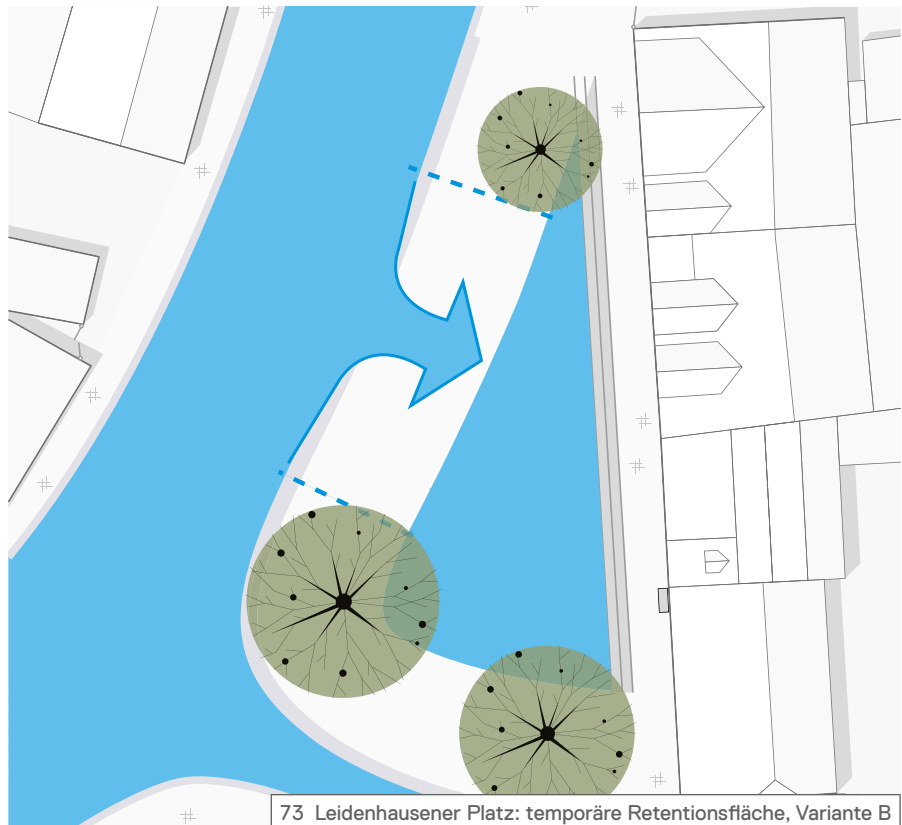
73 Leidenhausener Platz: temporäre Retentionsfläche, Variante B
